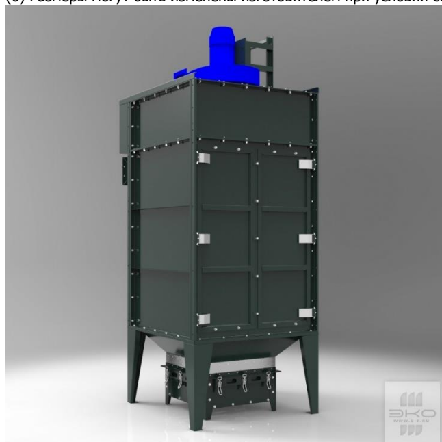
СРФ4К-ВЕНТ с выдвижным ящиком
